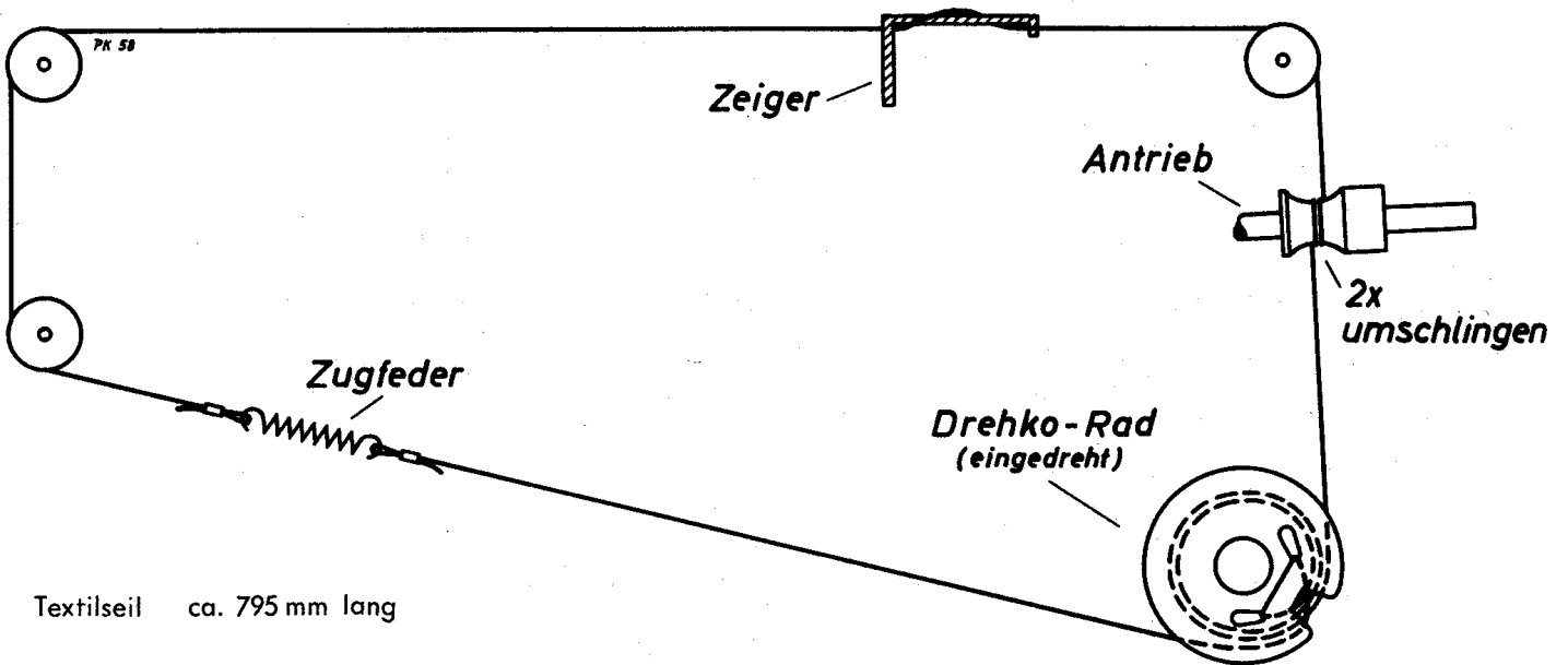
Schnurlaufführung TS 58 von der Lautsprecherseite gesehen
