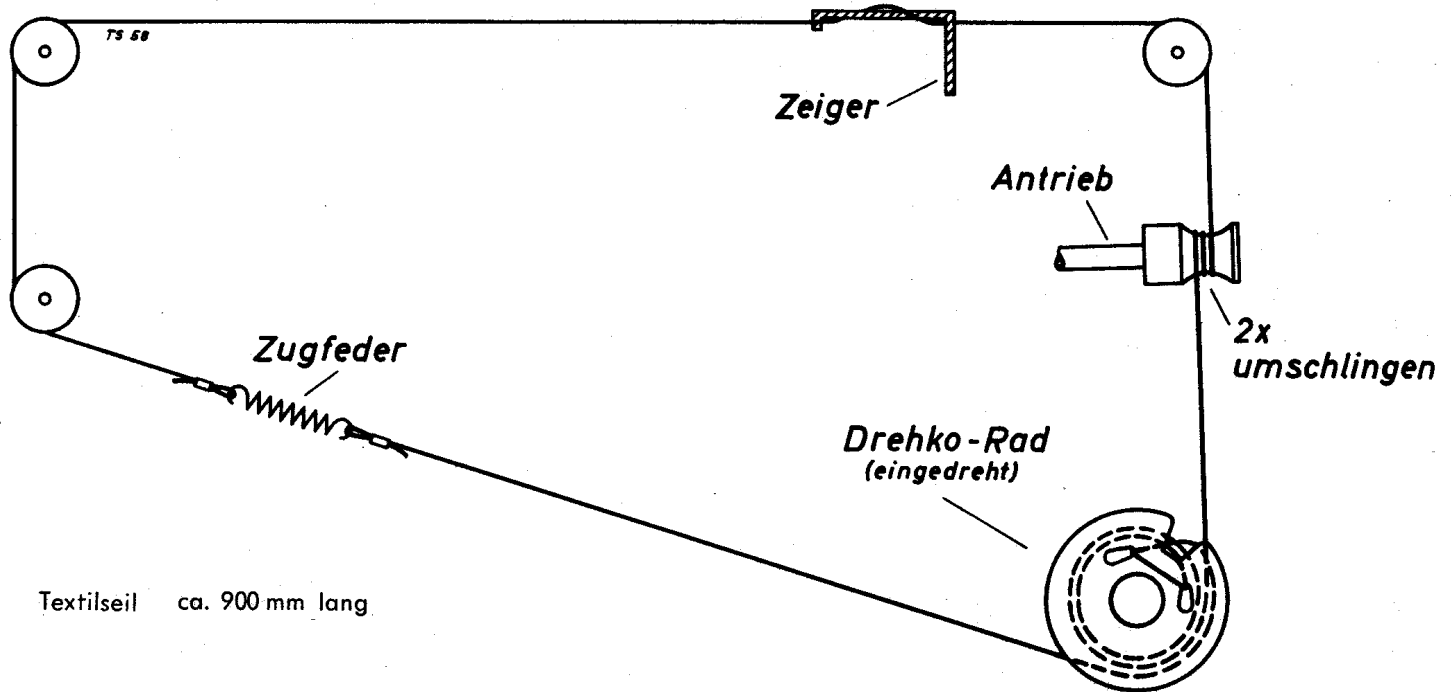
Schnurlaufführung TS 58 von der Lautsprecherseite gesehen
